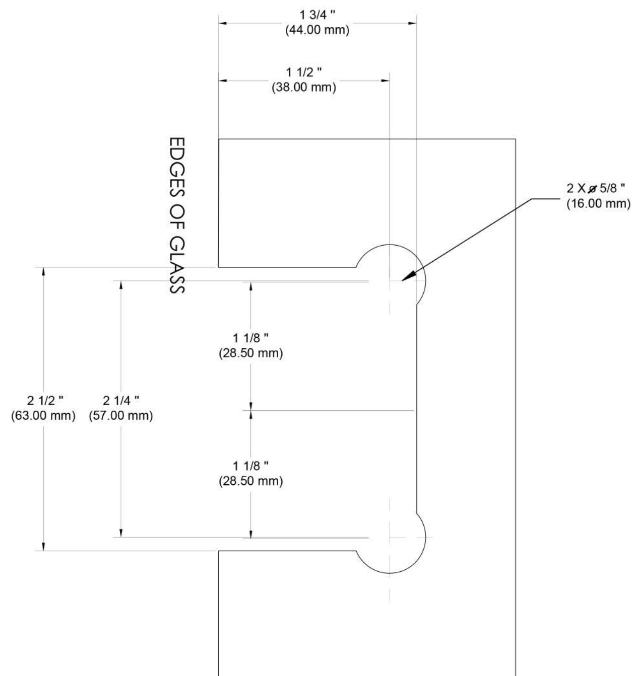
DOOR TEMPLATE
